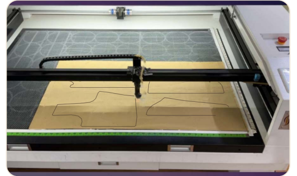
लेज़र बेड पर कपड़ा — सॉफ़्टवेयर फ़ाइल सीधे।
